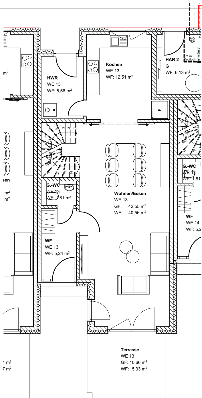
Erdgeschoss
