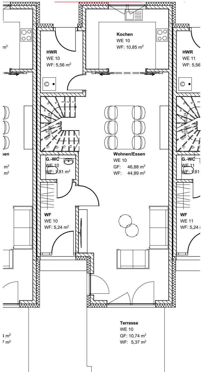
Erdgeschoss
