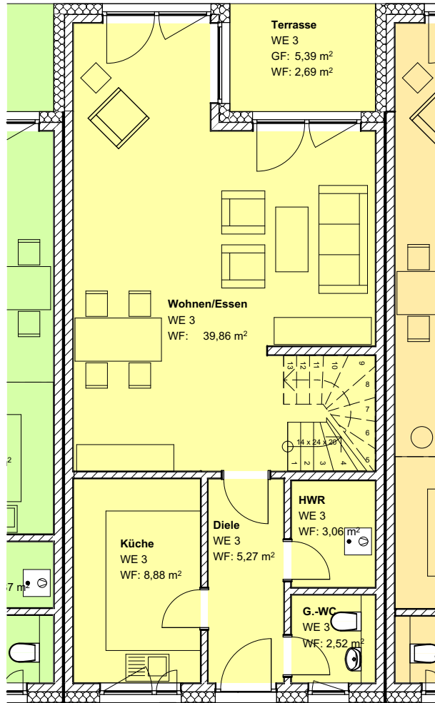
Erdgeschoss
